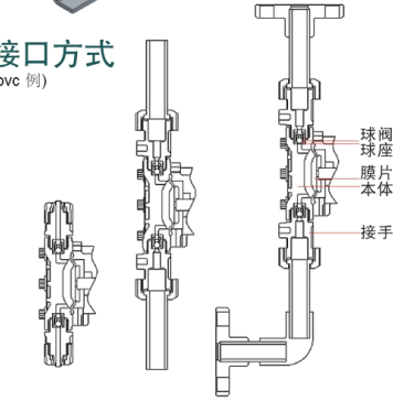
软管式 由令式 法兰式
